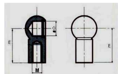
CAGE A ROTULE METALIQUE
