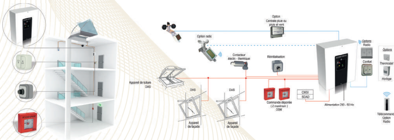
Schéma d'installation dans une cage d'escalier
