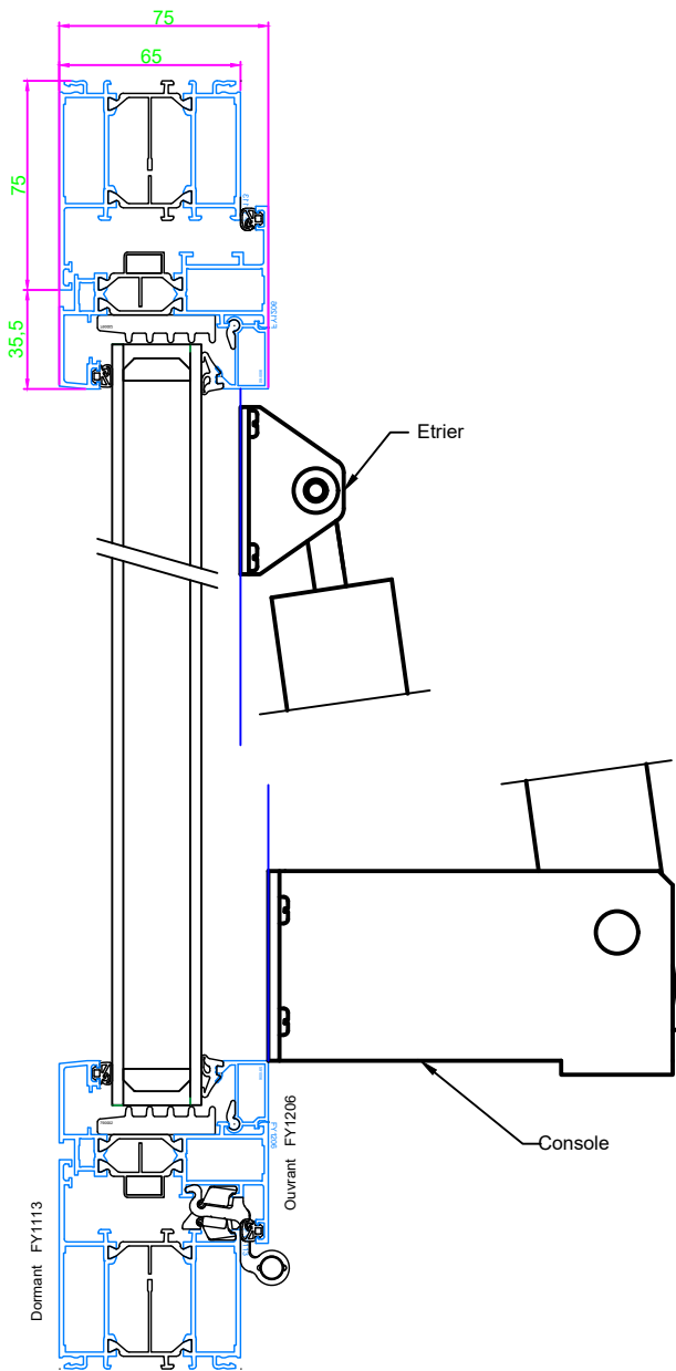
Coupe horizontale BB
