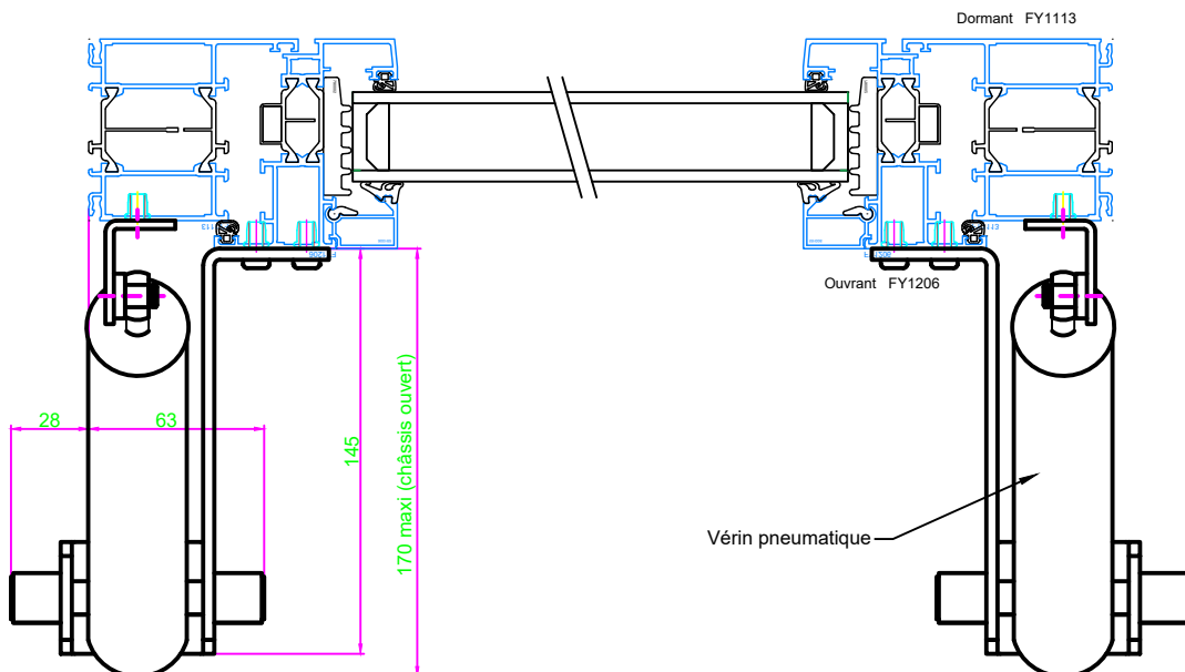
Coupe horizontale BB
